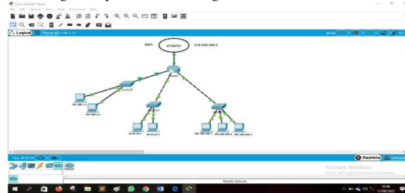
Gambar 3. Skematik Jaringan Usulan (Sumber : Data Pengolahan Pribadi)
