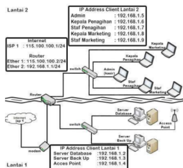
Gambar 2. Skematik Jaringan Berjalan (Sumber : PT BCA Multifinance)
