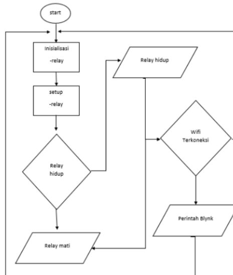
Gambar 3.2. Flowchart perangkat keras
