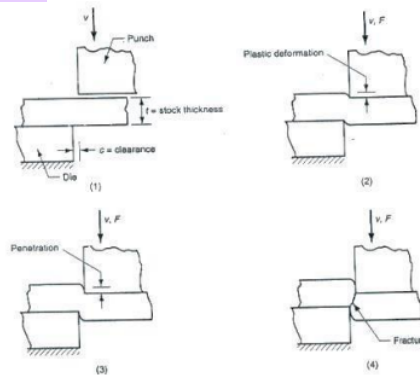
Gambar 12. Tahapan Pemotongan
