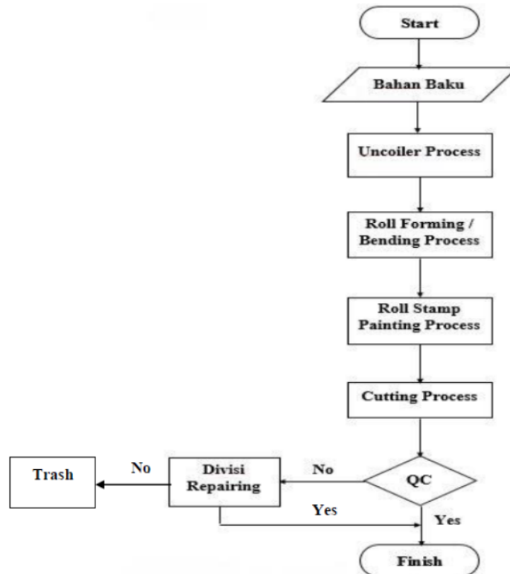
Gambar 1. Flowchart Proses Pembuatan reng baja ringan
