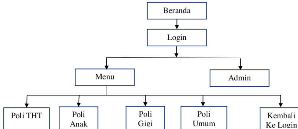
2 Gambar 2. Struktur Navigasi Hirarki Aplikasi
