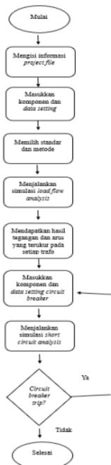
Gambar 1. Diagram Alur Simulasi
